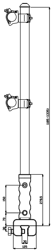
概略図
